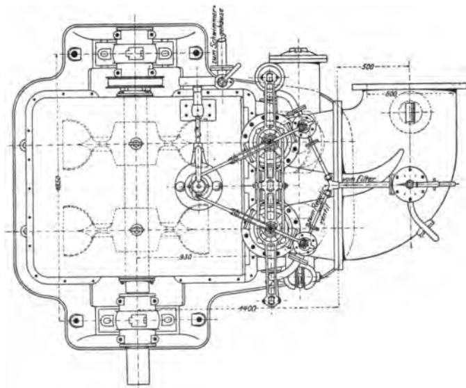
Fig. 66. Pelton-Turbine in Kubel bei St. Gallen.
